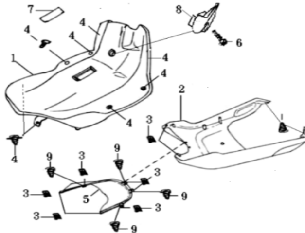
F17 Leg shield
