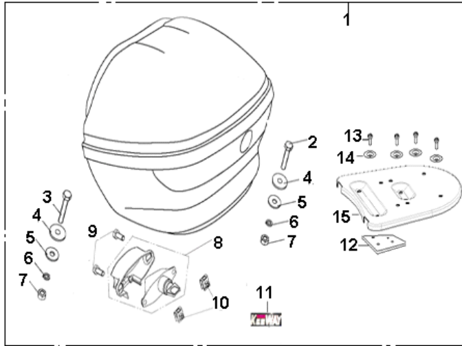
F13back box assy
