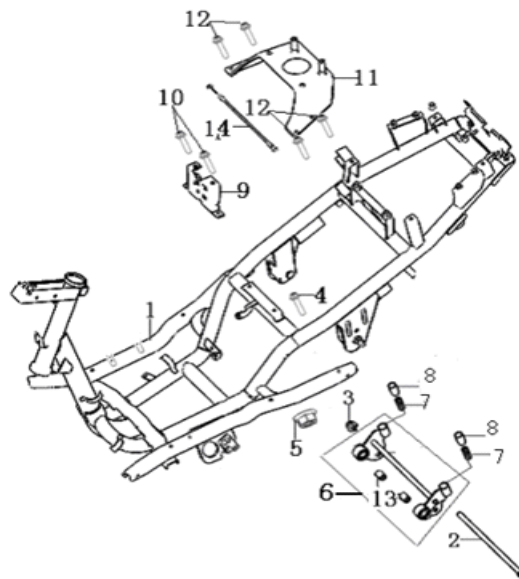
F11 Frame body
