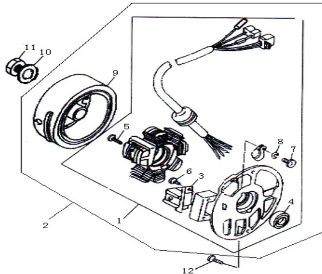
E11 MAGNETO ASSY
