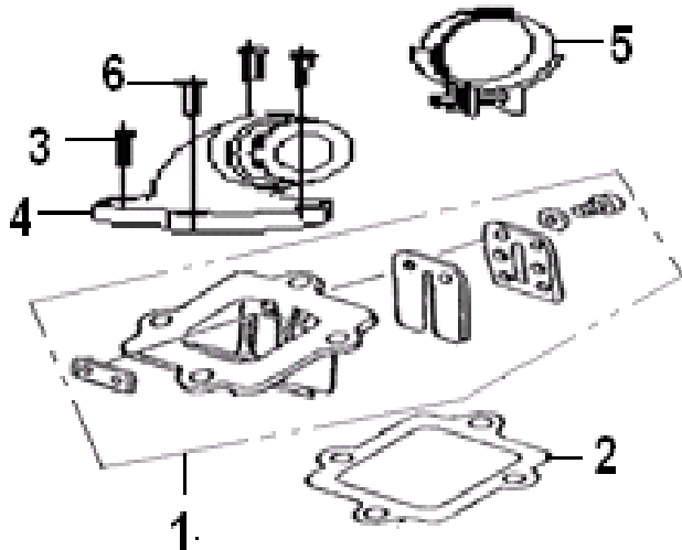
E10 REED VALVE ASSY
