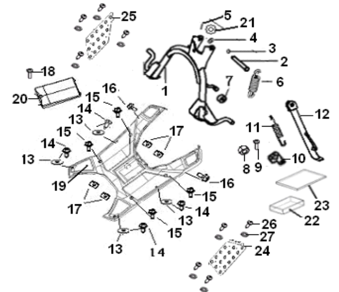
F18 Footrest / Stand
