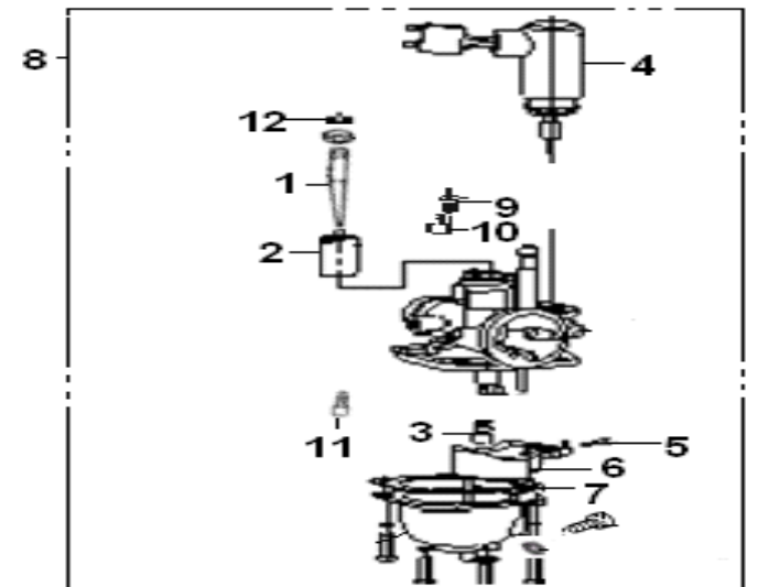
E12 CARBURATOR ASSY
