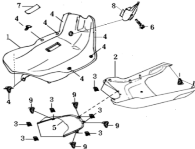
F17 Leg shield
