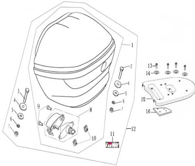
F13back box assy
