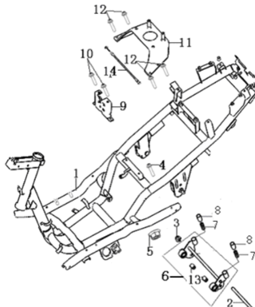
F10 Frame body
