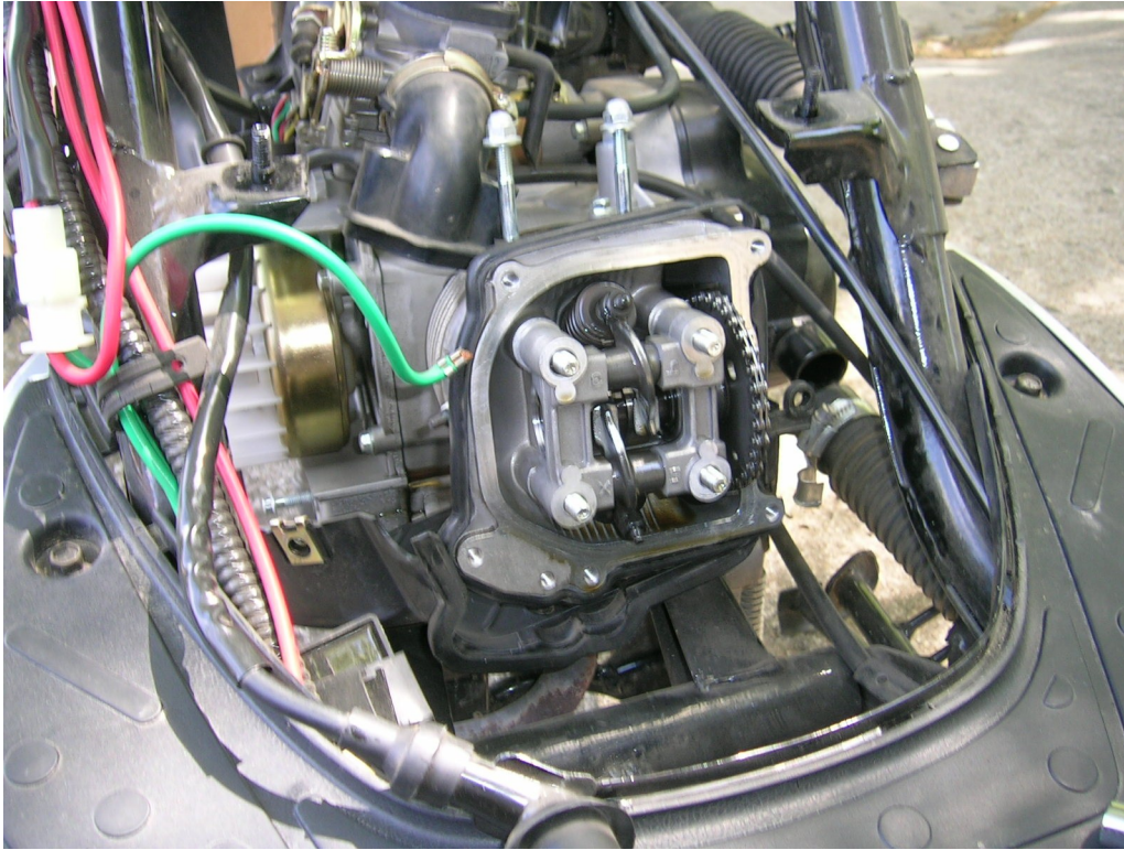
Fig. 6. Remove camshaft caps (before)
